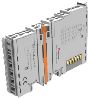
Pulse output module,2 port,24V
